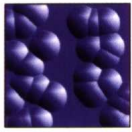
分子
