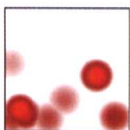
有丝分裂
