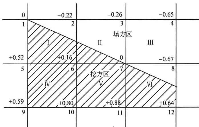
图 1-8 施工高程计算图
