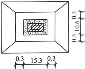
图 1-6 基坑平面图(单位：m)
