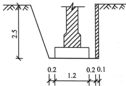
图 1-12 沟槽示意图(单位: m)
