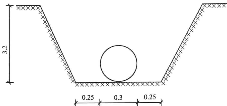
图 1-2 开挖管道沟槽断面图 (单位: m)
