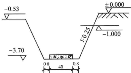
图 1-11 基坑示意图(单位: m)
