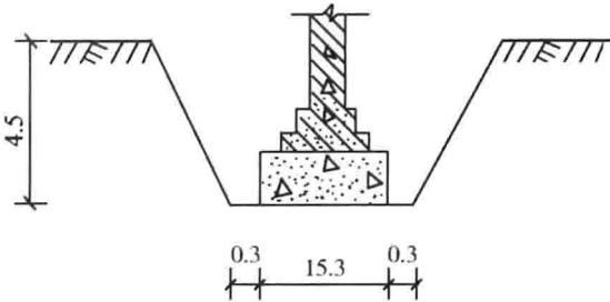
图 1-5 基坑断面图(单位：m)
