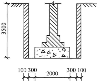
图 1-4 沟槽断面图
