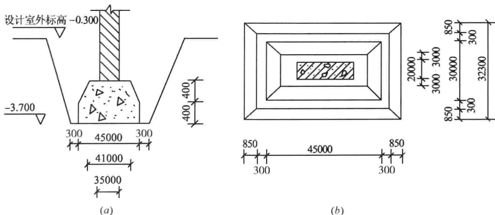
图 1-13 基坑示意图
