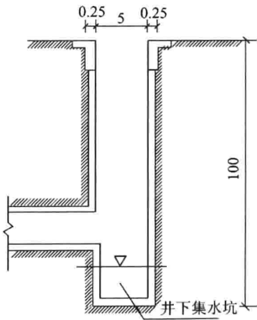
图 1-10 竖井断面图(单位: m)
