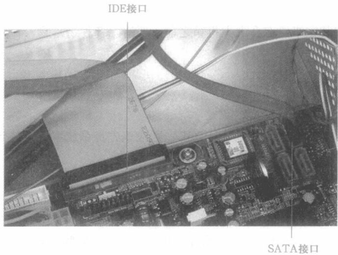
图 1-1-16 微型计算机外部存储器设备数据传输线连接方法
