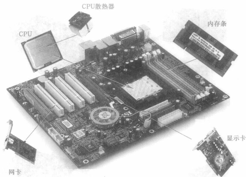
图 1-1-15 微型计算机的系统主板及主要部件的安装位置
