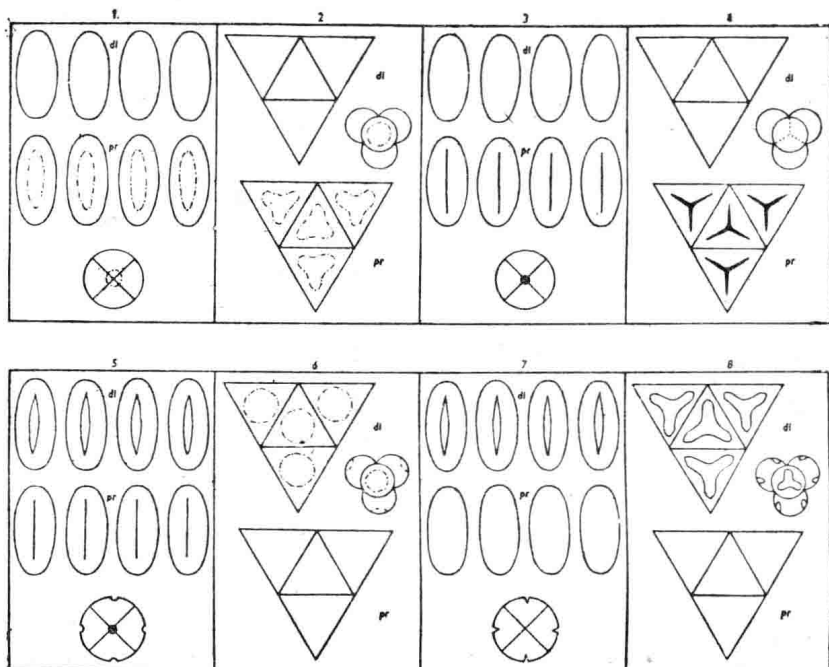
图1 1—14.花粉和孢子四分体
