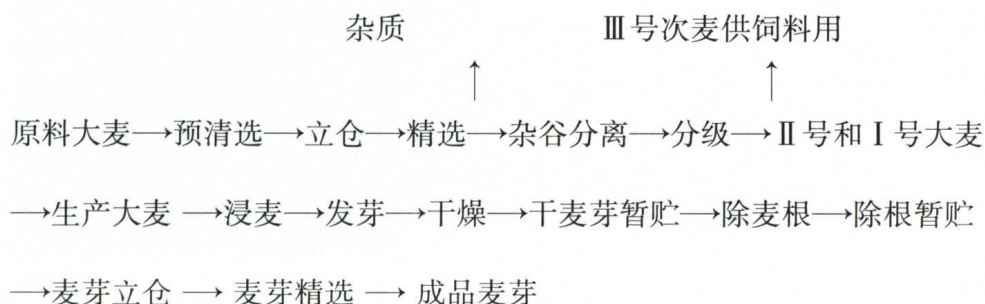
图 1-7 麦芽生产工艺流程图
