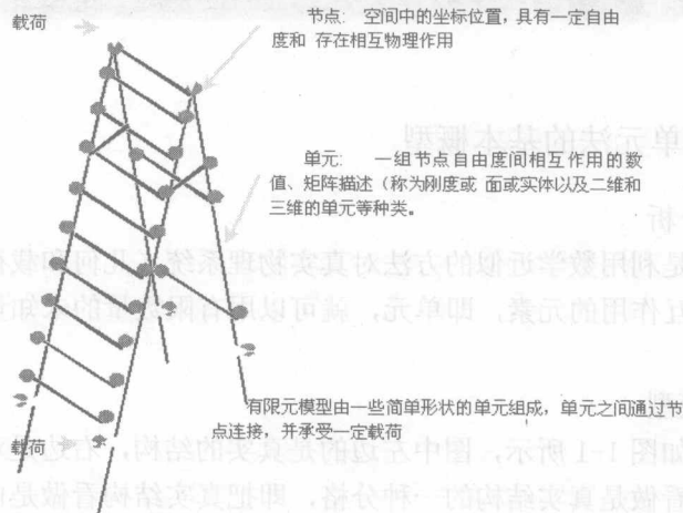
图 1-3 节点和单元
