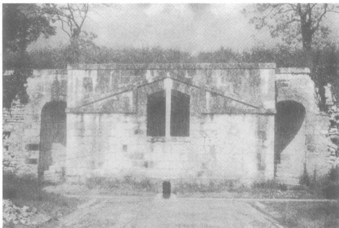
布鲁阿日堡垒（滨海夏朗德省），建于 17 世纪， 军官们的厕所（AGL 照片）。
