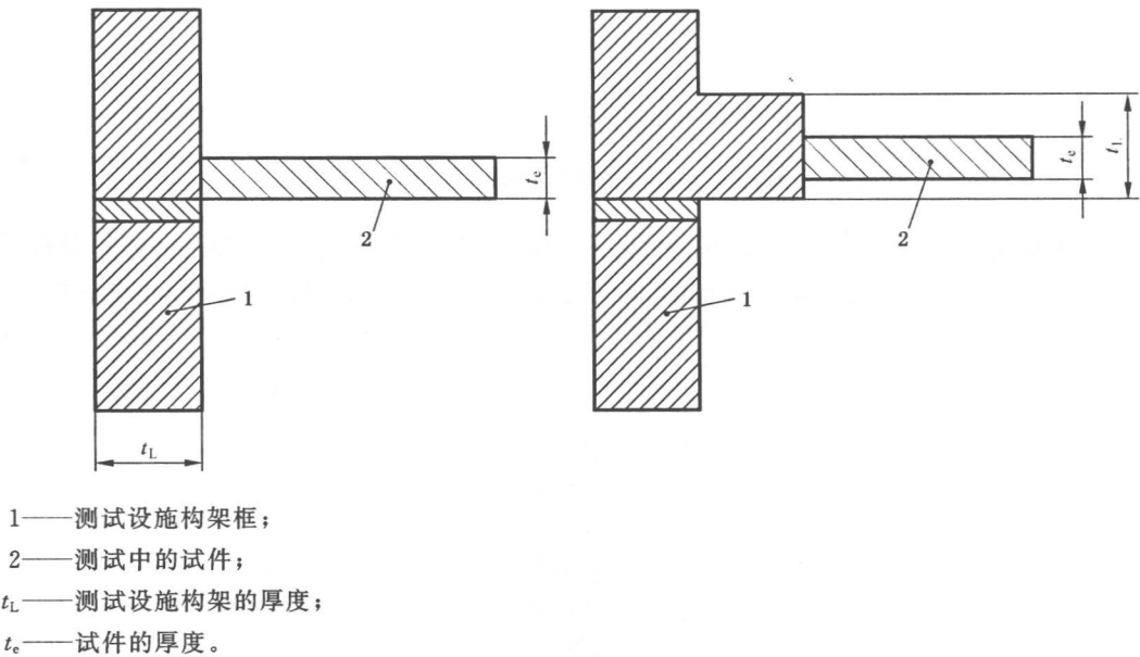
图 D.2 计算构件单位面积质量的示意图
