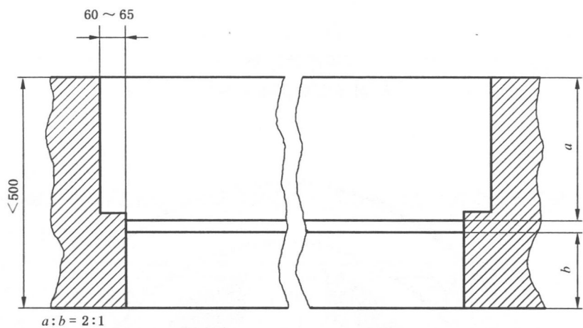
图 1 安装玻璃的测试洞口的尺寸, 水平剖面
