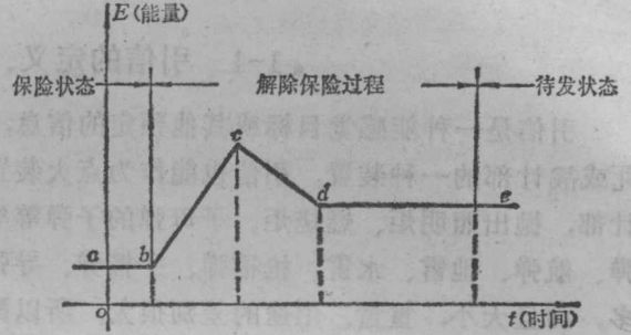
图 1-1 典型的引信解除保险过程
