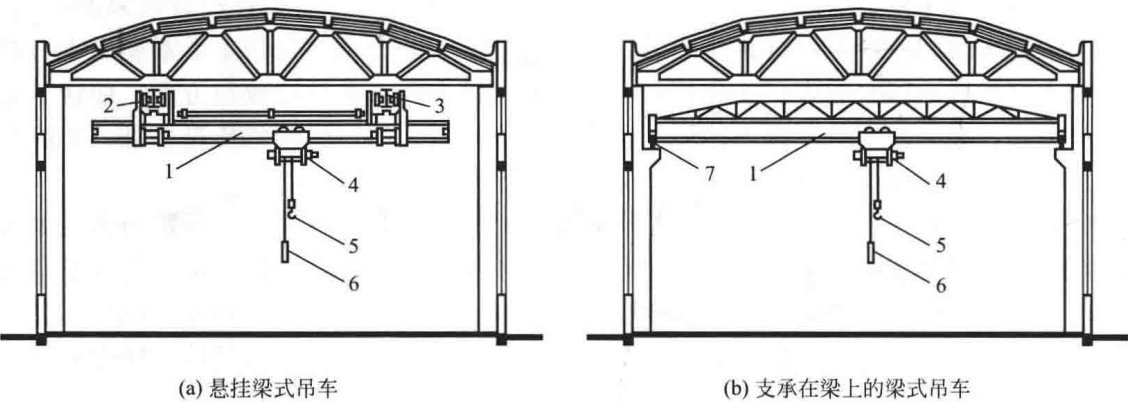
图 1.5 梁式吊车
