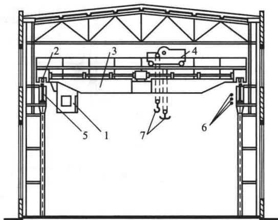
图 1.6 桥式吊车
