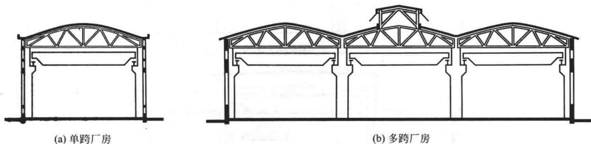
图 1.1 单层厂房
