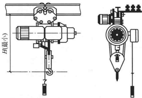
图 1.4 单轨悬挂式吊车
