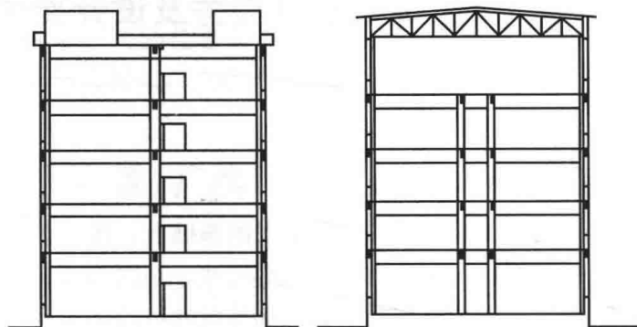
图 1.2 多层厂房
