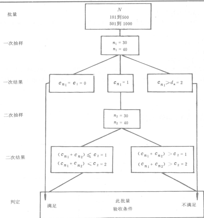
图2 二次抽样图
