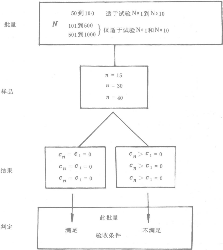
图1 一次抽样图
