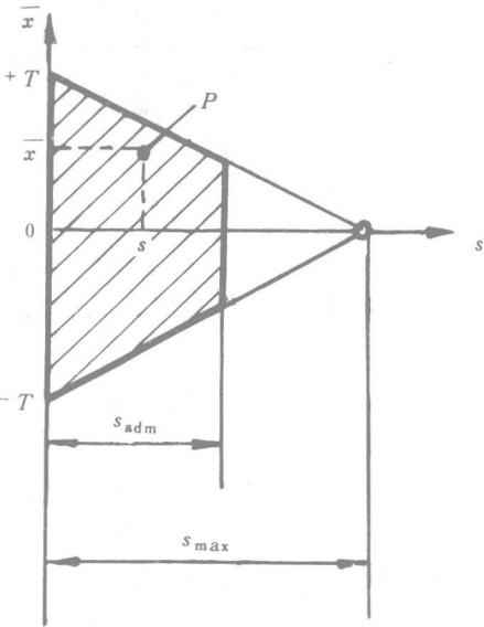
图 3 验收梯形
