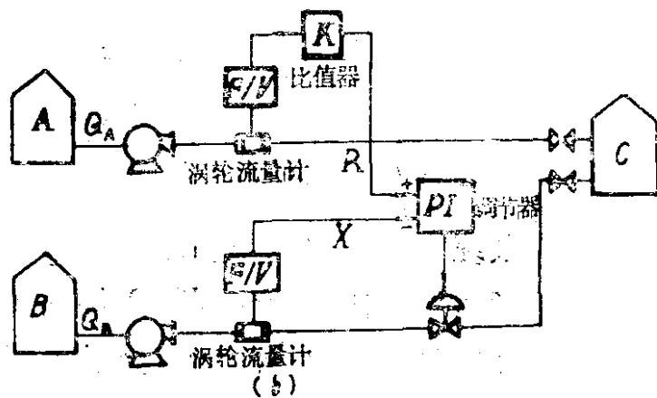
图1-2 负反馈说明示例
