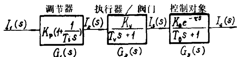
(b) 串接环节
