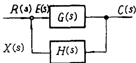
(c) 反馈系统
