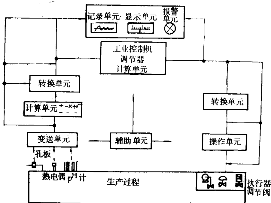
图 1-1 仪表调节系统的组成
