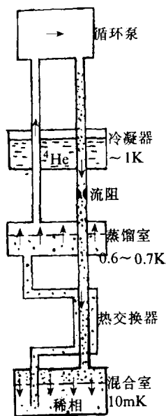
图 0-4 稀释制冷机
