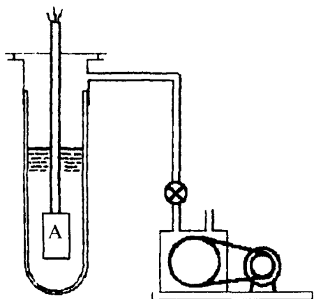
图 0-3 减压降温恒温器
