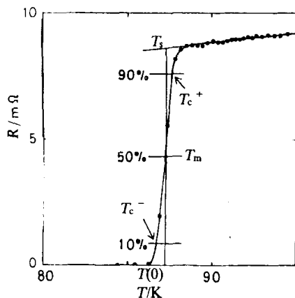
图 1-1 R-T 曲线
