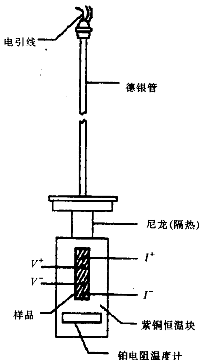
图 1-2(a) T_c 测试探头示意图
