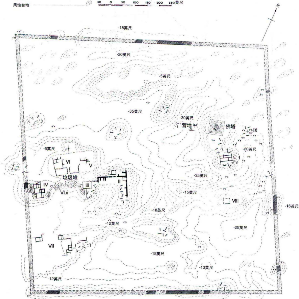
图16 楼兰LA古城平面图
