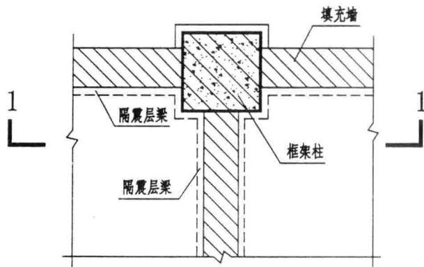
①/6 框架边柱节点(边梁与柱对中)
