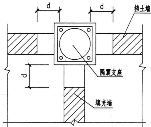
3-3
