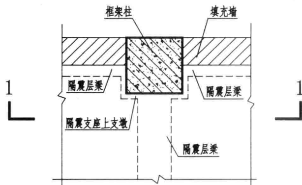
1/6 框架边柱节点 (边梁与柱不对中)
