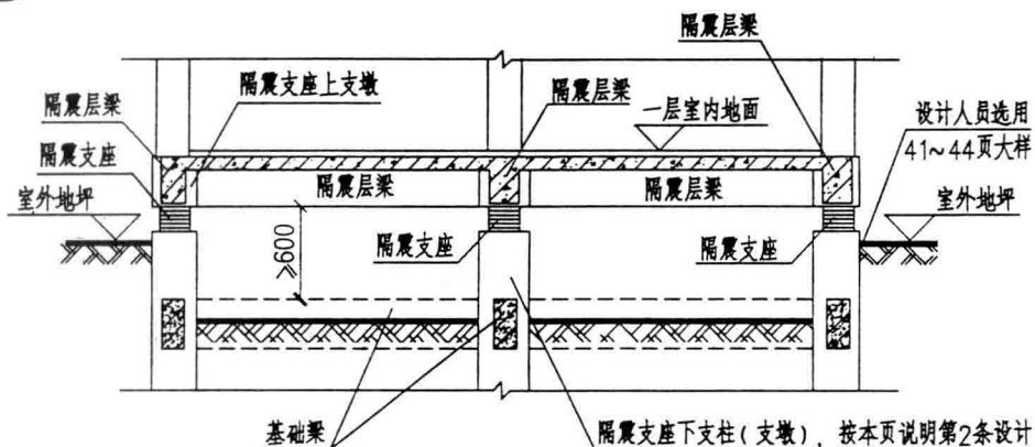
1-1 (无地下室)
