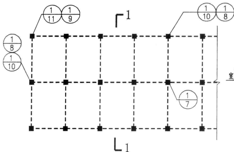
框架结构隔震支座平面布置示意
