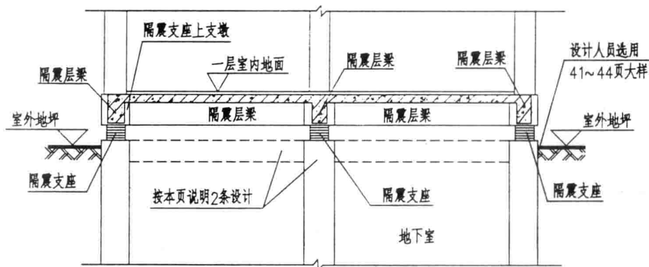
1-1 (有地下室)
