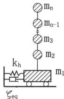
图1 隔震结构计算简图
