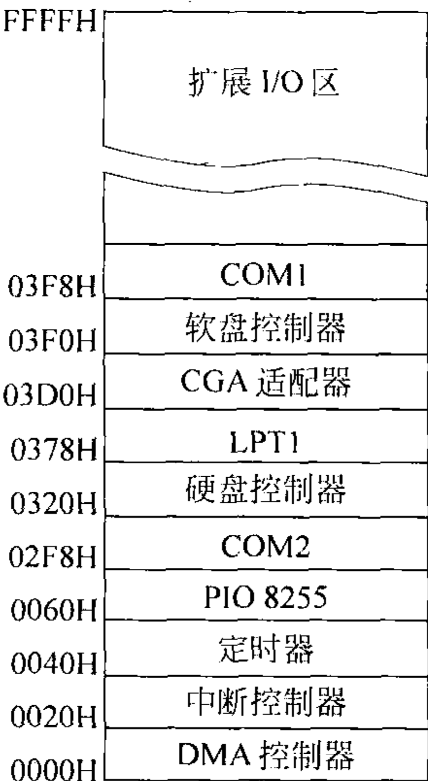
图 1-6 PC 的 I/O 映像区
