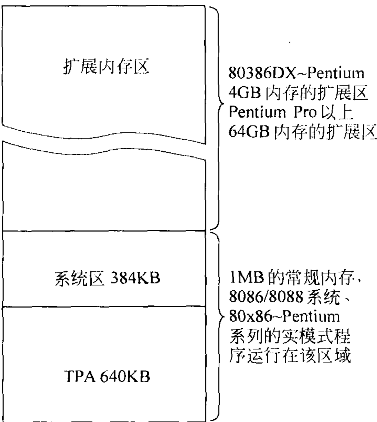
图 1-5 PC 的内存存储器映像区
