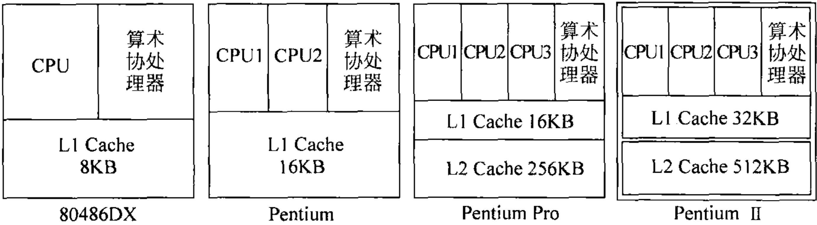
图 1-4 几种微处理器的粗略结构
