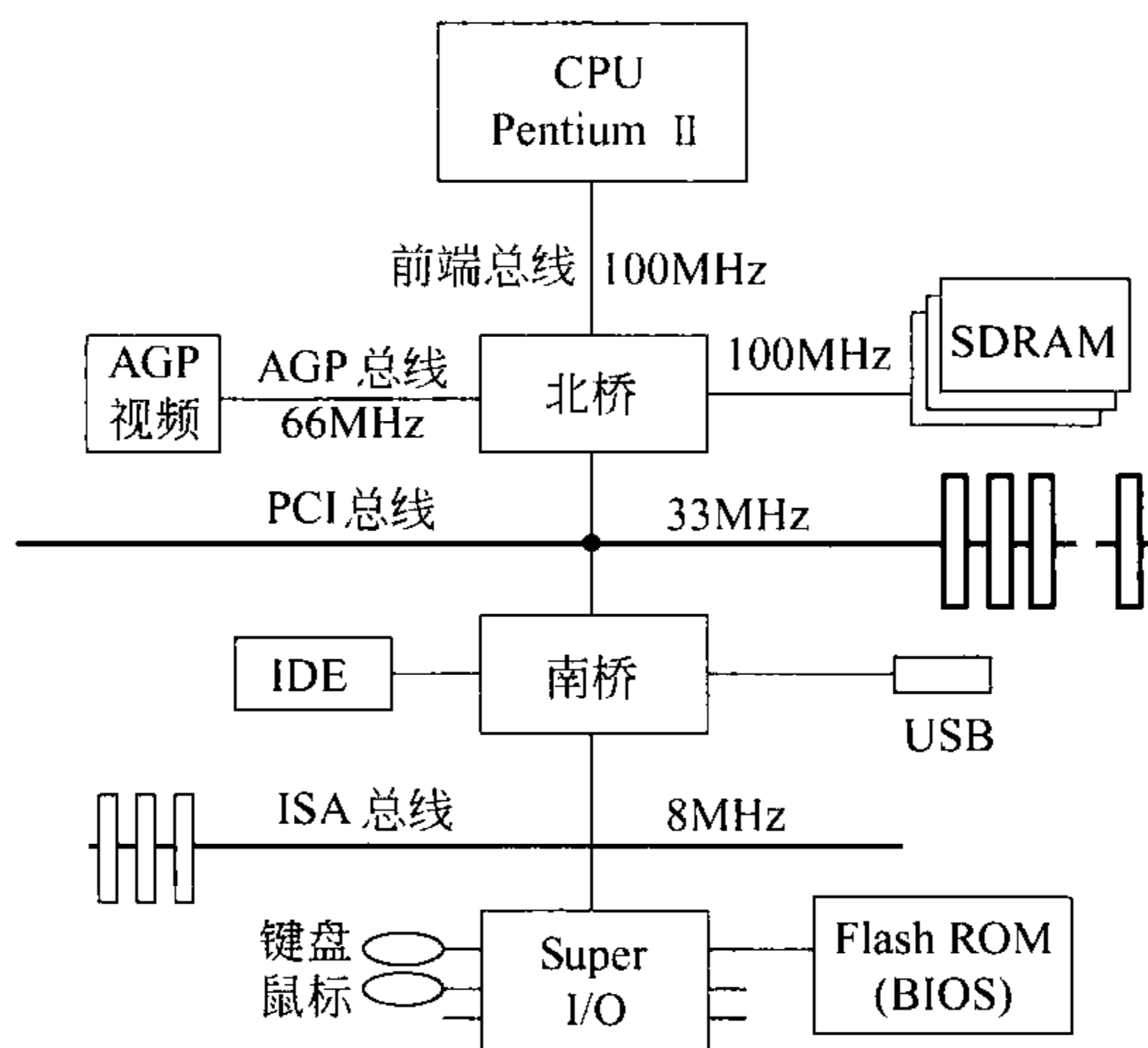
图 1-7 基于 PCI 总线的微型计算机结构
