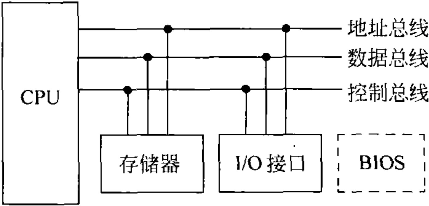
图 1-2 微型计算机的基本结构
