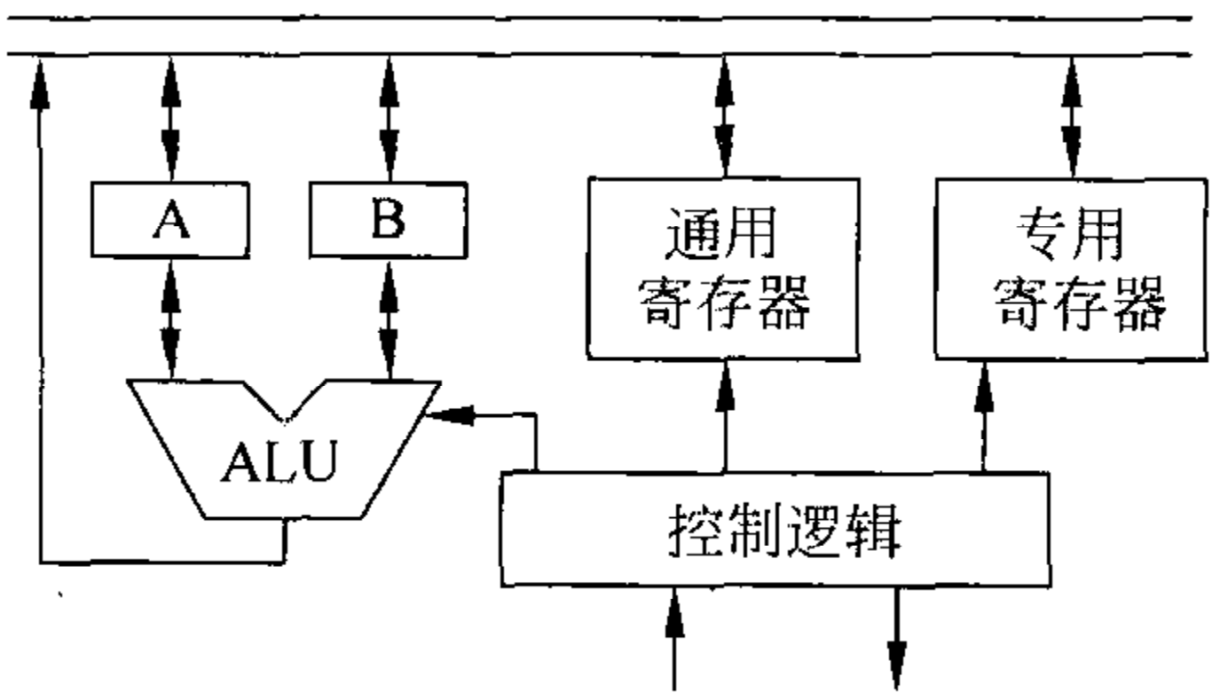
图 1-3 中央处理器的基本单元
