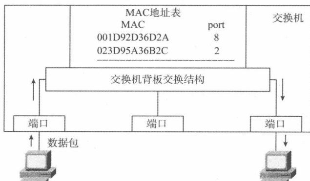
图 1-1 交换机结构
