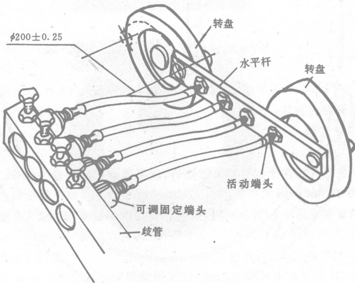
a 挠曲疲劳试验机
