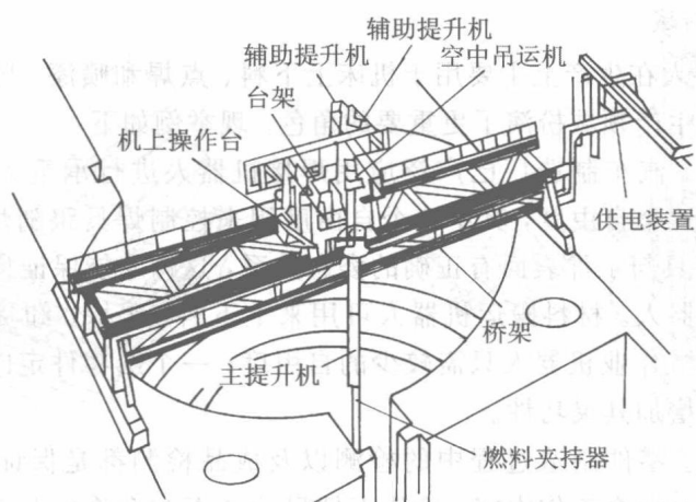
图 1.9 沸腾水式反应堆燃料自动交换机
