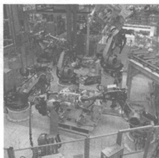
图 1.2 汽车焊接生产线上的机器人
