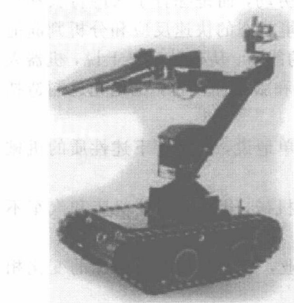
图 1.3 排爆机器人
