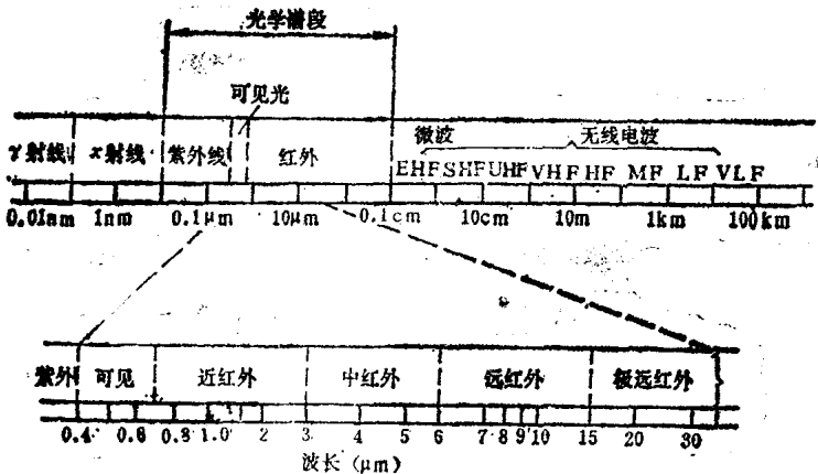
图0-1 电磁频谱
