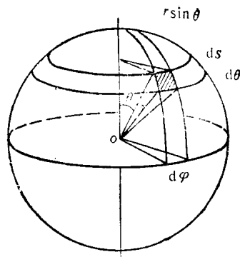
图1-2 角度增量对应的立体角
