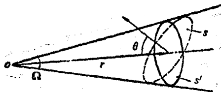
图1-4 与射线束成一定角度的平面的立体角
