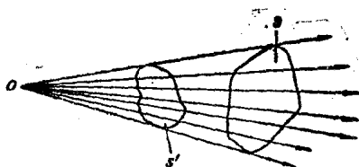
图1-3 射线束围成的立体角
