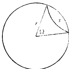
图1-1 立体角的概念
