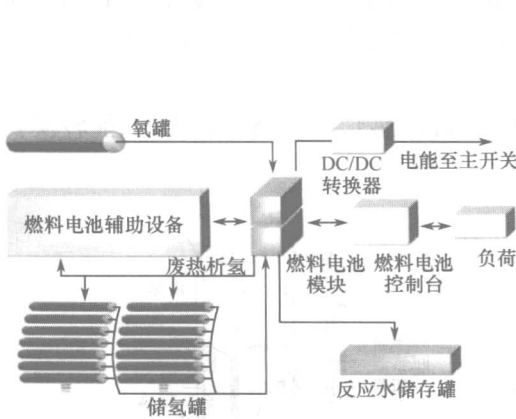
图 1-7 FC/AIP 的构成
