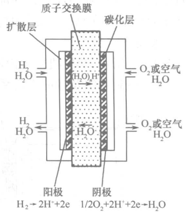
图 1-8 PEMFC 燃料电池原理
