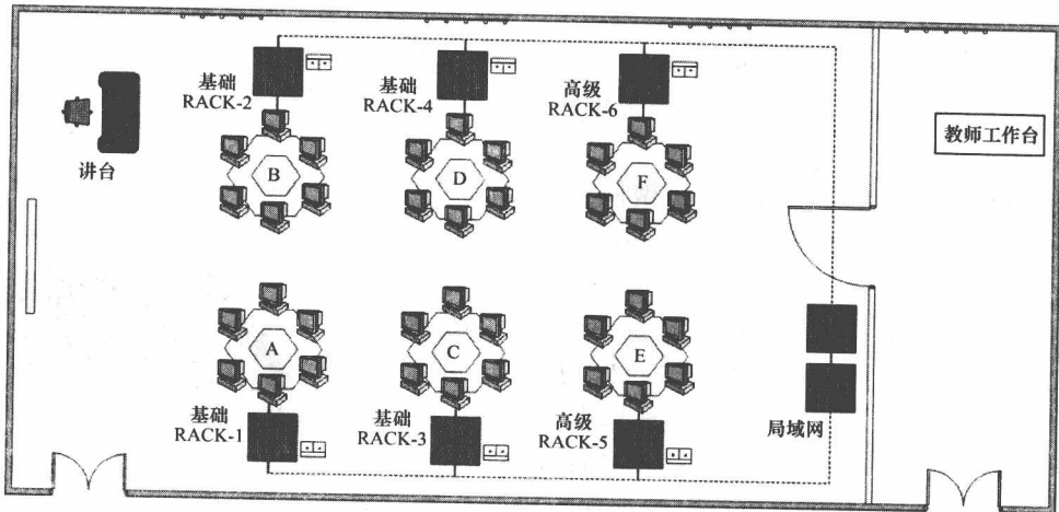
图1-5 实验室的布局
