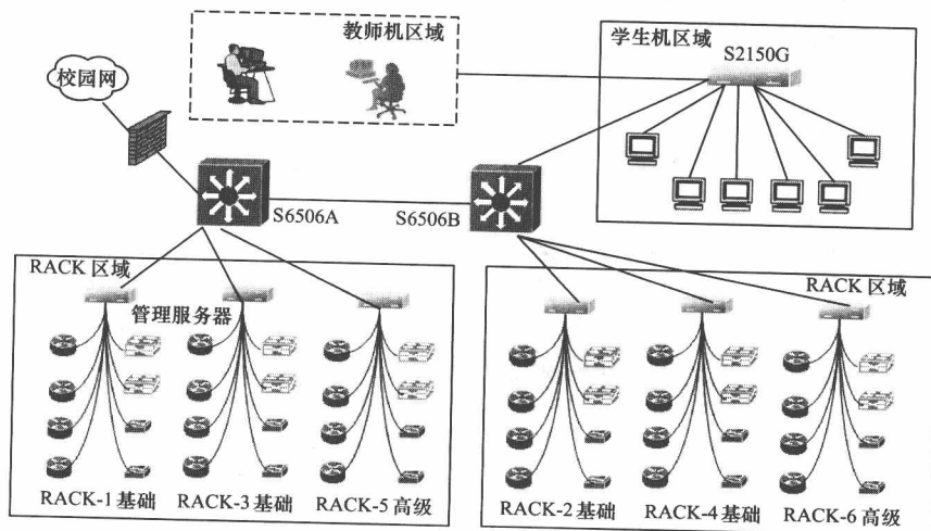
图 1-1 网络实验室拓扑结构
