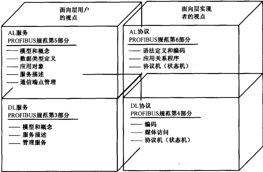
图 2 DL/AL 服务和协议部分分开的概念
