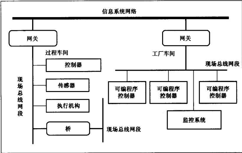
图 1 一般的现场总线网络
