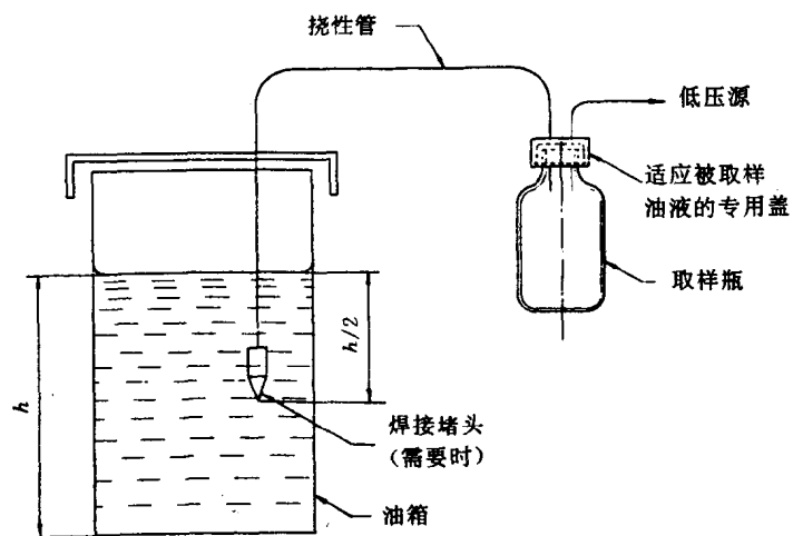
图 2 油箱取样器的典型示例
