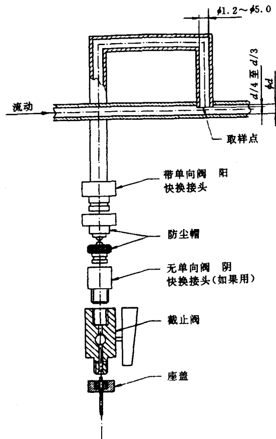
图 1 现场型取样器的典型示例
