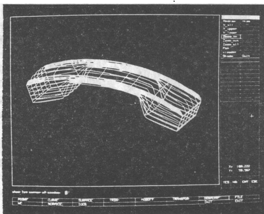
图3 电话听筒的曲面造型
