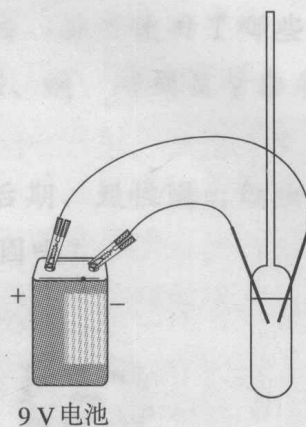
图 1-7 电解污水的微型实验
