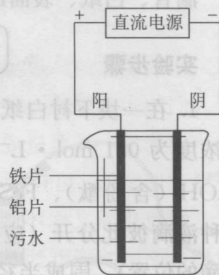
图 1-6 电解污水实验
