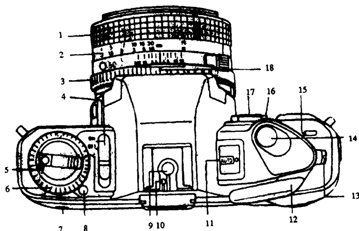
图 1-4 照相机的构造
