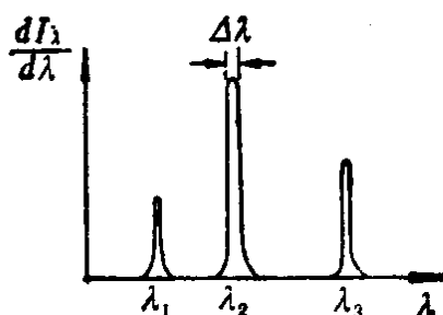
图 0-2 线光谱
