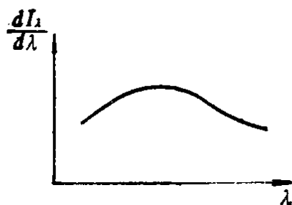
图 0-1 连续光谱
