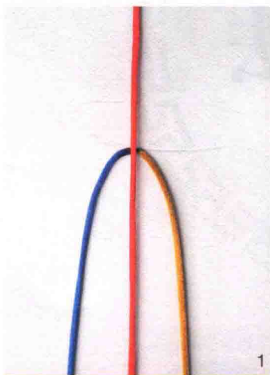
1. 将两条线烧连成一条线，再同另一条线如图中所示的样子摆放。
