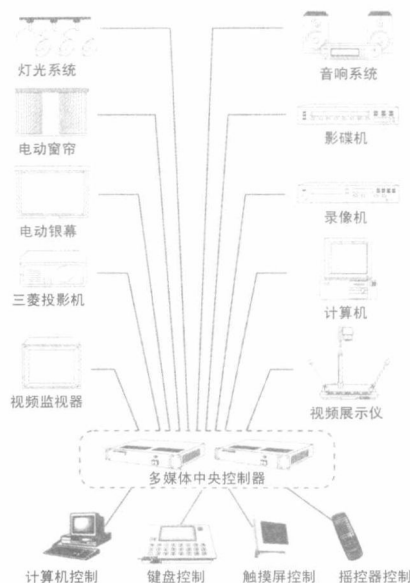
多媒体控制系统结构图示
