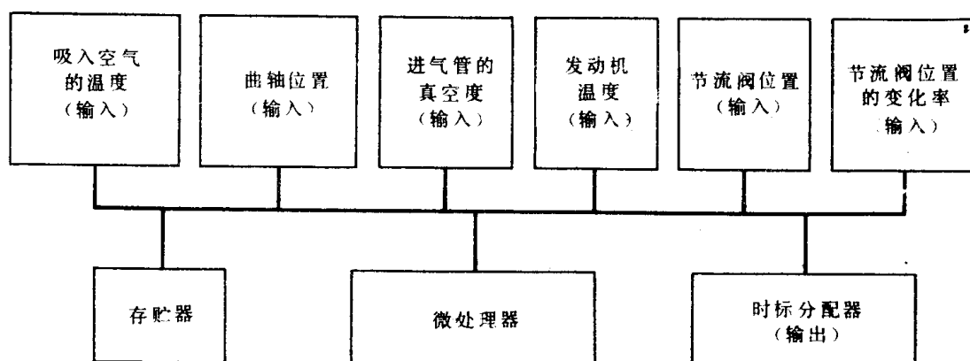
图1-6 汽车的点火定时系统框图
