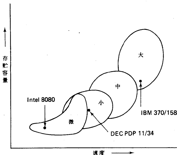
图1-3 计算机速度与存储容量的关系
