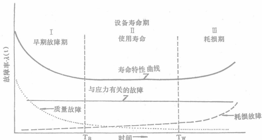
图 1.1 故障率函数曲线
