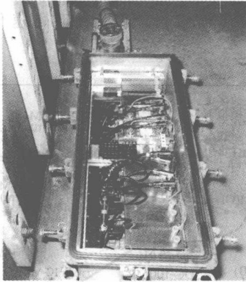
图 1.4 在人井内设置的中继器
