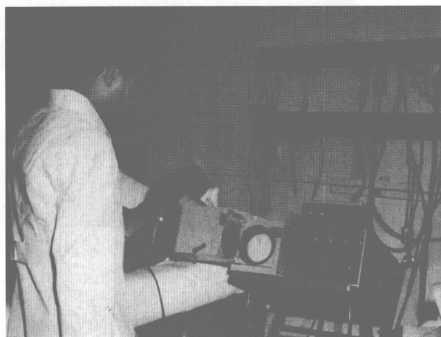
图 1.8 早期应用 Polaroid 照相机记录超声心动图的 M 型超声心动图仪
