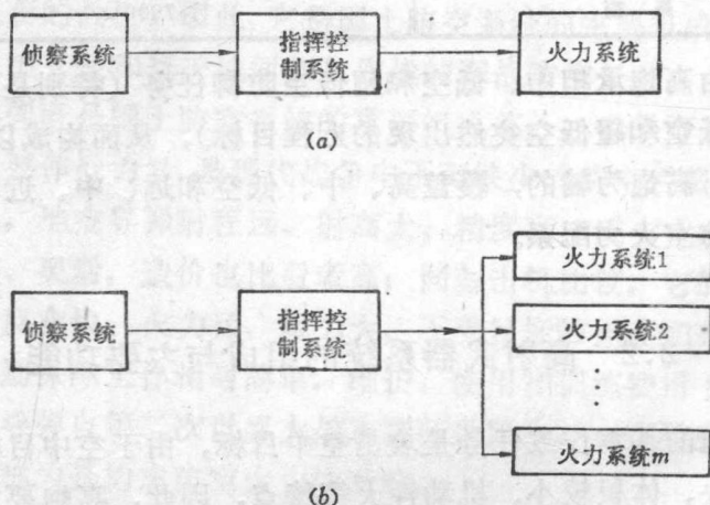
图2.2 高射武器系统组成结构框图
