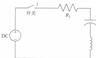
图 1-5 RLC 电路
