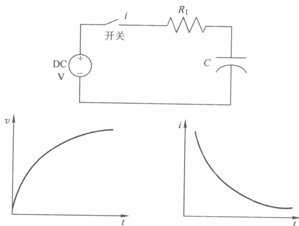
图 1-4 RC 电路和暂态特性
