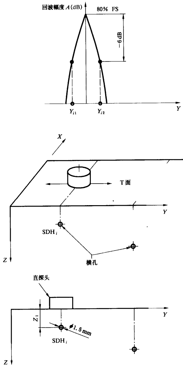
图 3 直探头的声束测量
