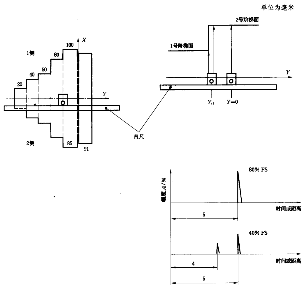
图9 斜探头在1号阶梯面上测得的声束半横截面宽度
