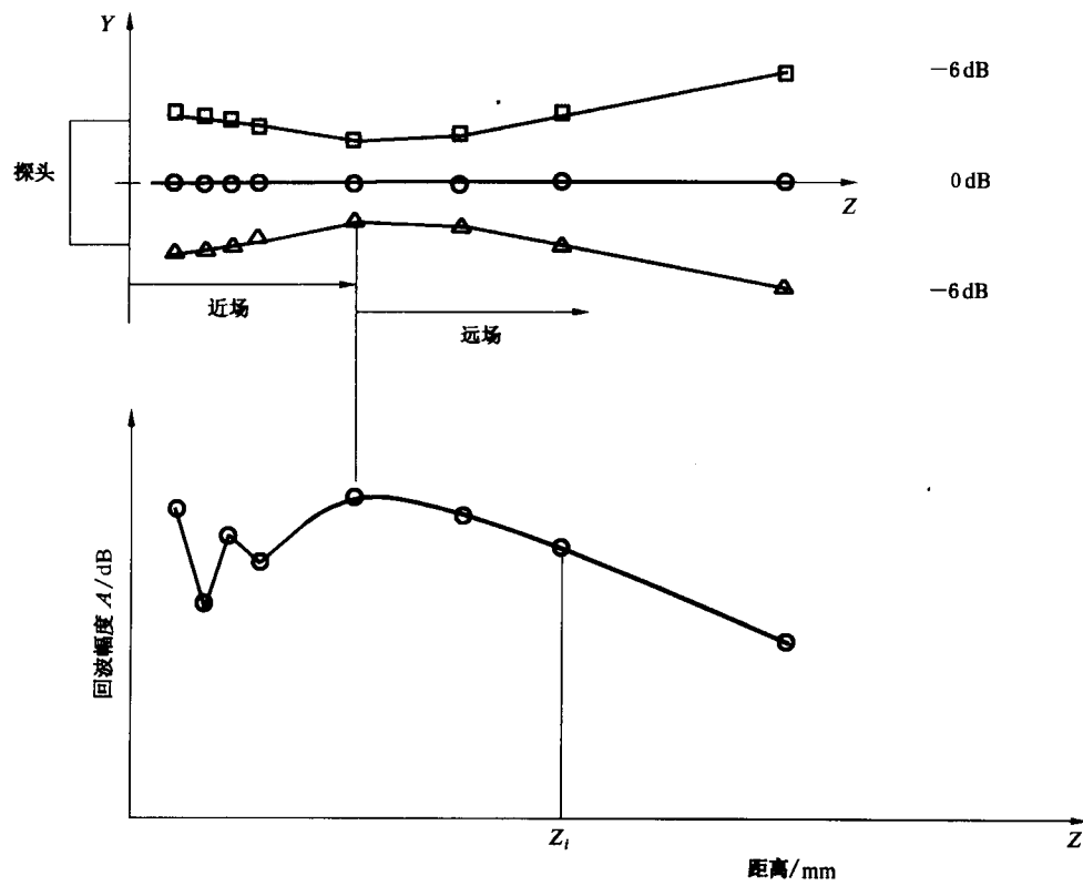
图 4 直探头的声束轮廓和幅度分布
