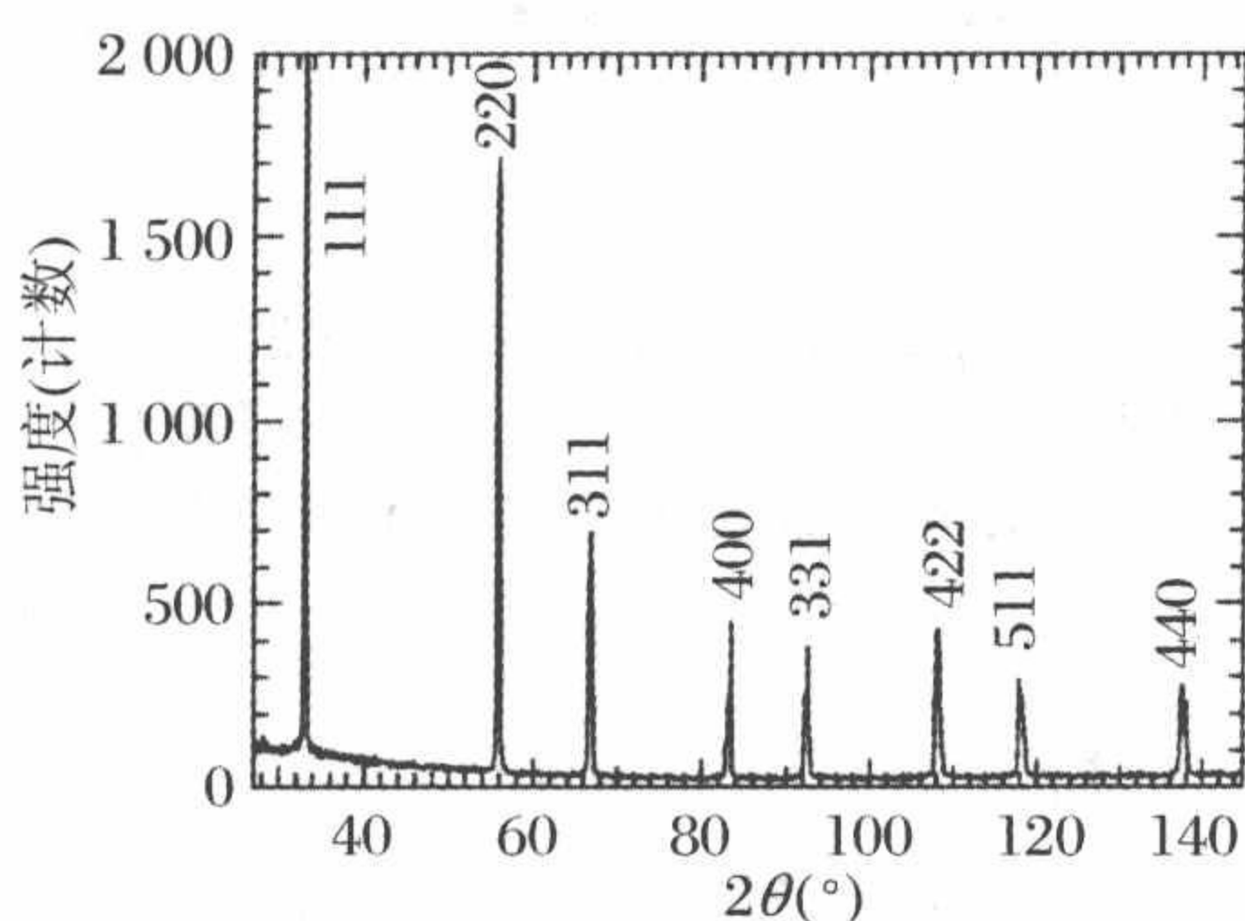
图 1.2 已指标化的多晶硅的粉末衍射图样(用 Co K_\alpha 测得)
