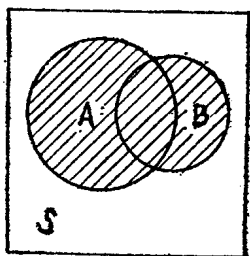
图 1-2 (a) 集合 A \cup B ；
