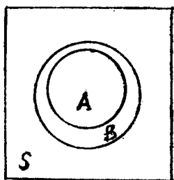
图 1-1 文氏(Venn)图
