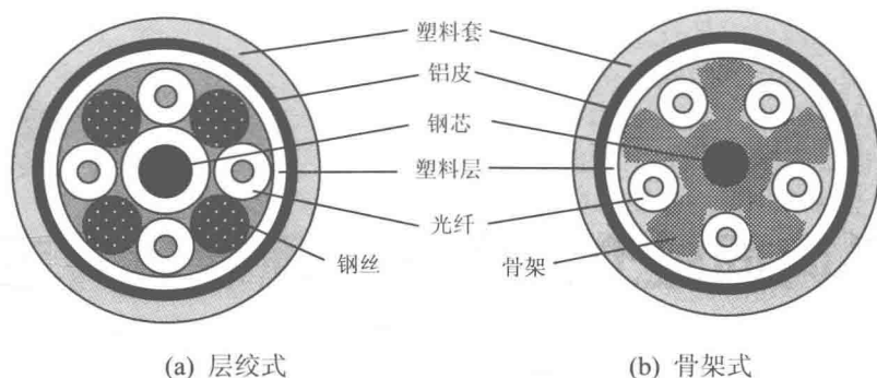
图 1.0 光缆示意图
