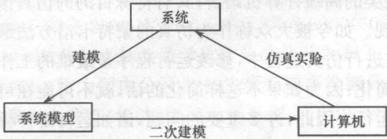
图 1.2 仿真三要素
