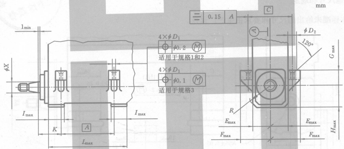
图 2 2 型架装直列式喷油泵
