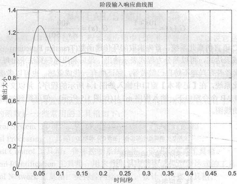
图 1.6 MATLAB 仿真程序的阶跃输入响应图
