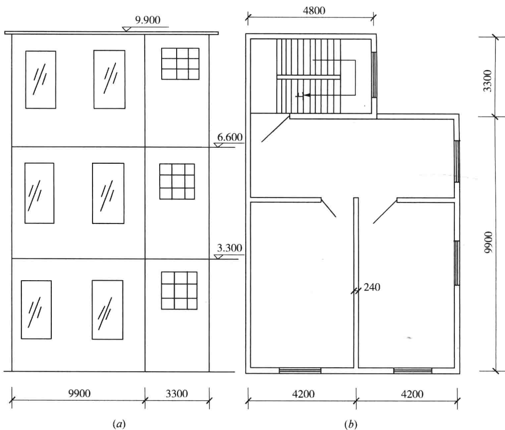
图 1-5 某别墅示意图 (a)东立面图；(b)二、三层平面图
