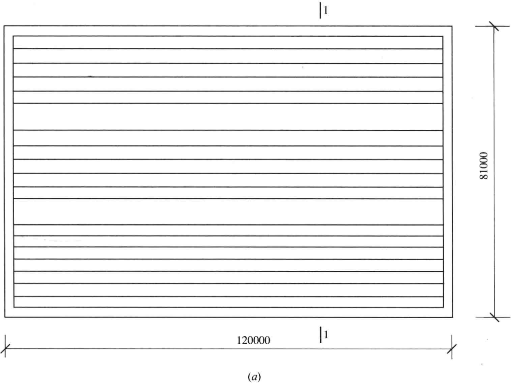
图 1-6 某体育馆看台示意图(一) (a)平面图
