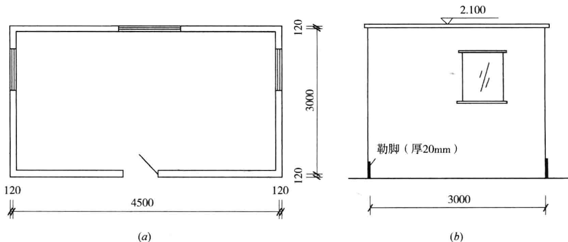
图 1-2 单层建筑物示意图
