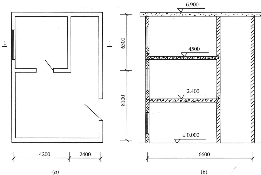
图 1-4 单层建筑物带部分楼层示意图
