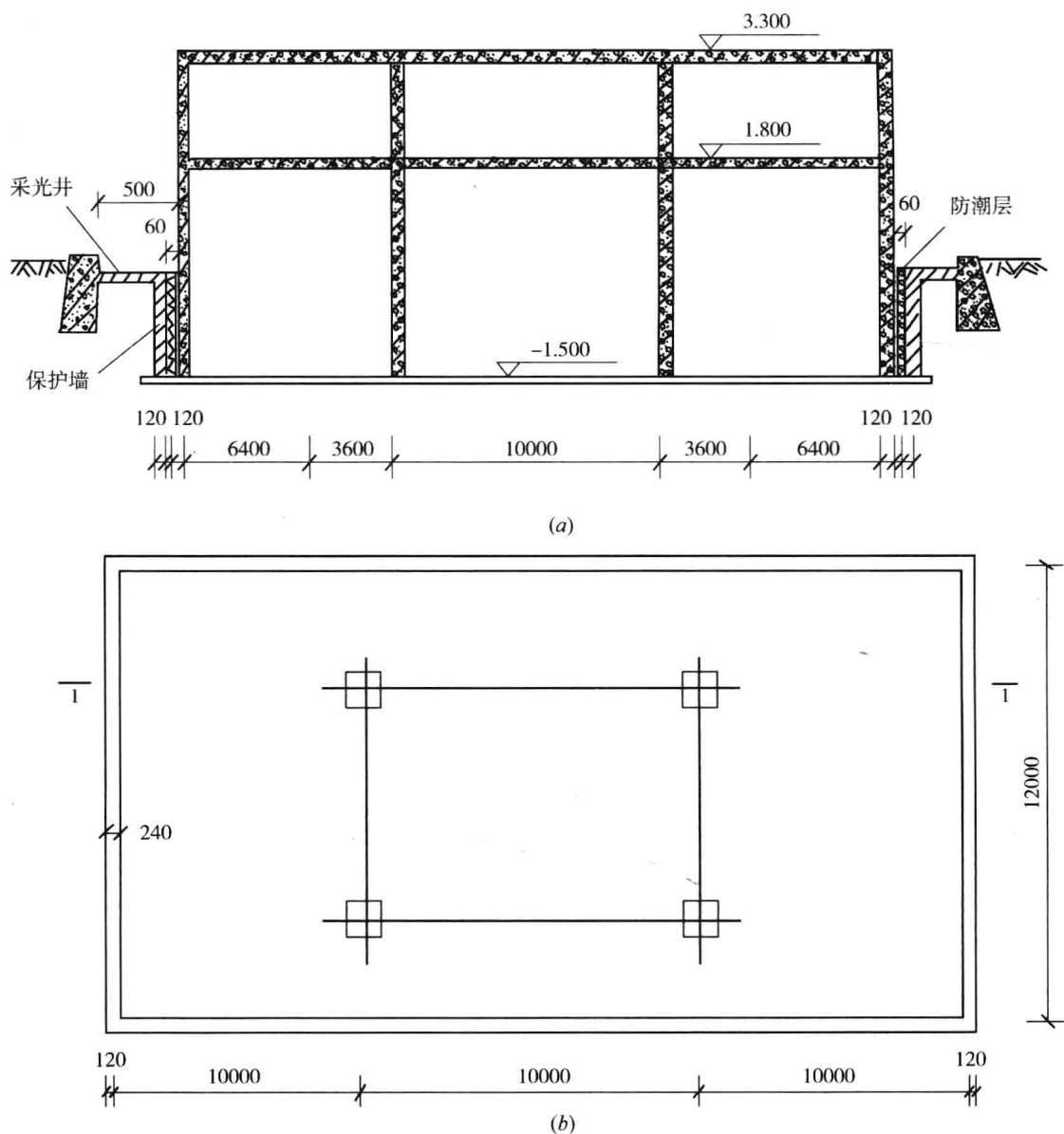
图 1-8 某商店示意图 (a)剖面图；(b)平面图
