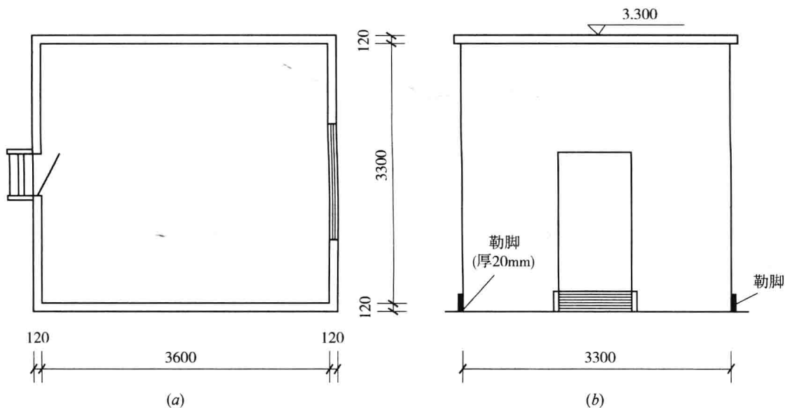
图 1-1 单层建筑物示意图 (a)平面图；(b)东立面图
