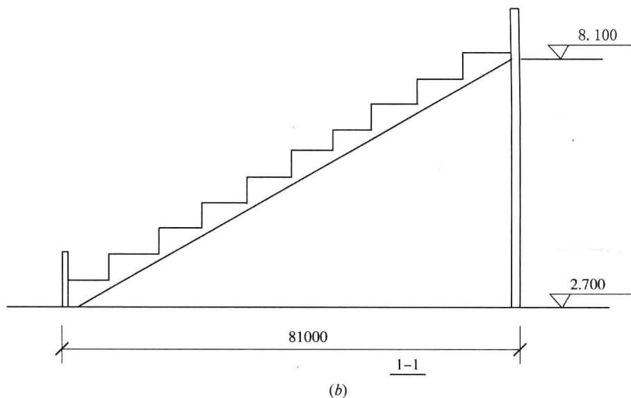
图 1-6 某体育馆看台示意图(二)
