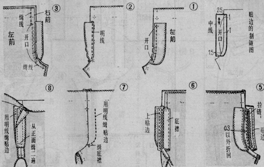
8. 上拉链B
