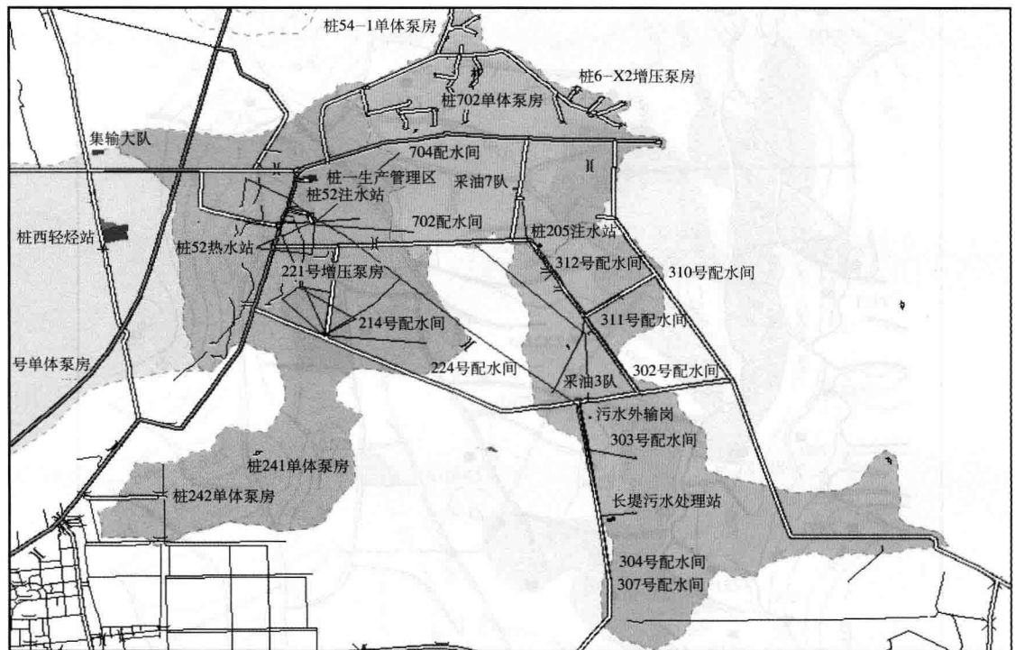
长堤油田注水系统管网分布图 (桩西采油厂地质研究所编制, 2005年)
