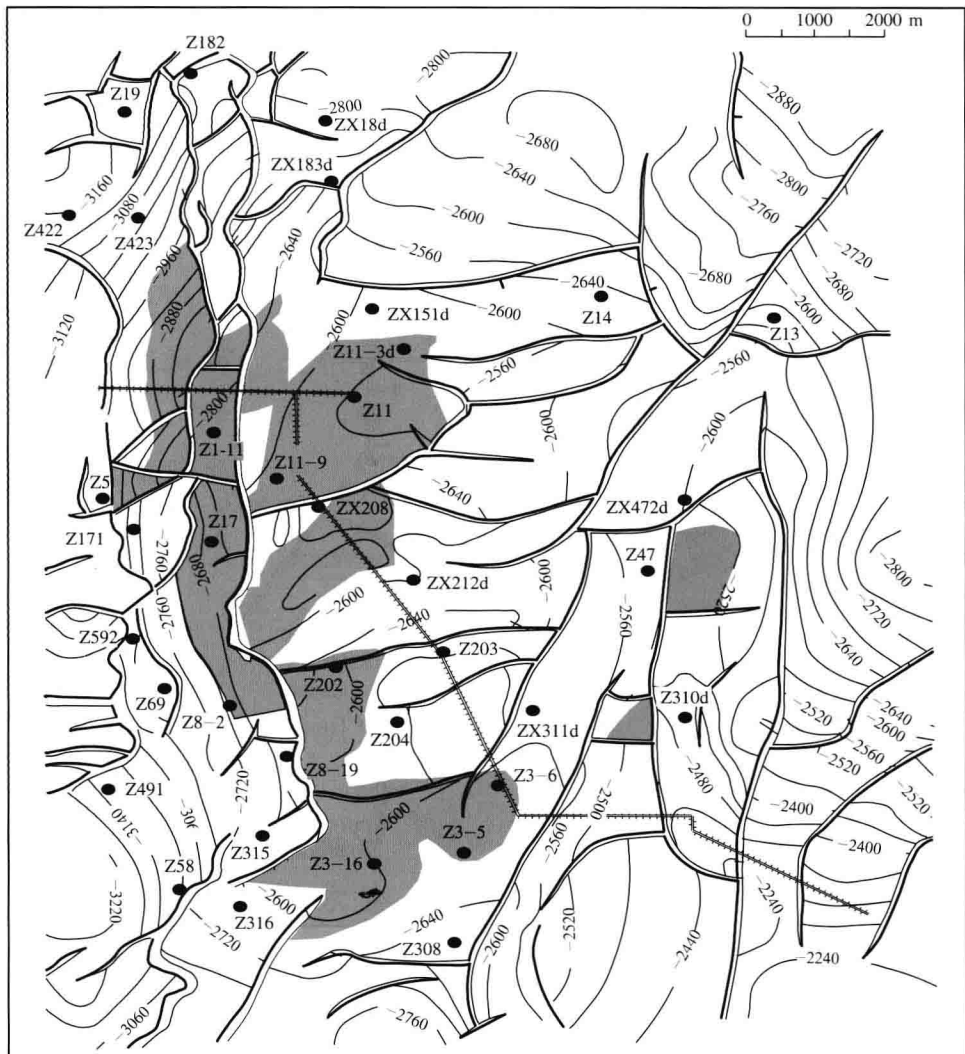
长堤油田构造井位图（桩西采油厂地质研究所编制，2005年）
