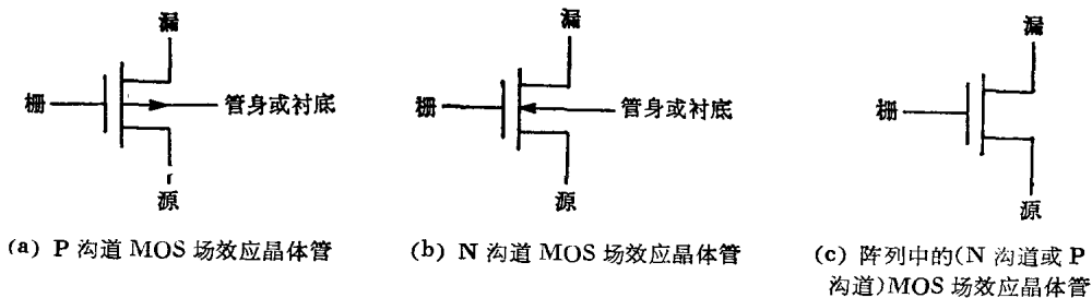
图 1-2 MOS 场效应晶体管的符号
