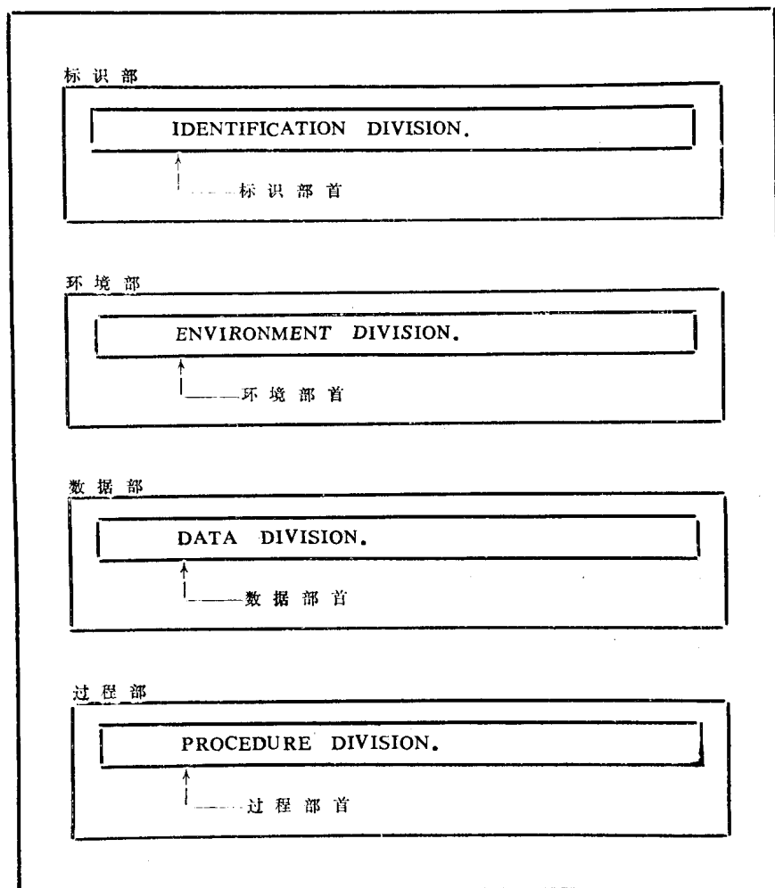
图3 COBOL 源程序的结构
