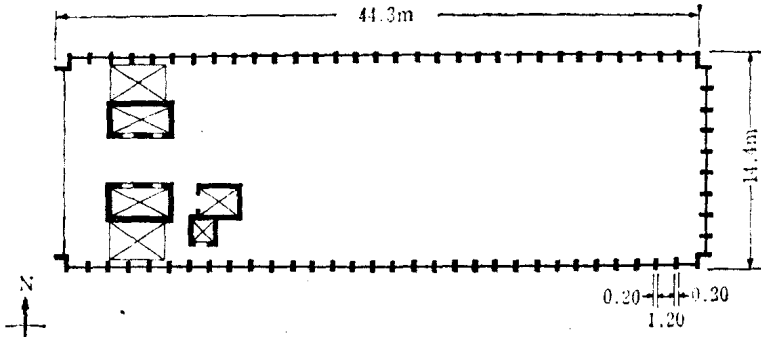
(b) 平面图(2)
