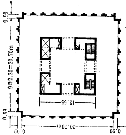
(a) 平面图
