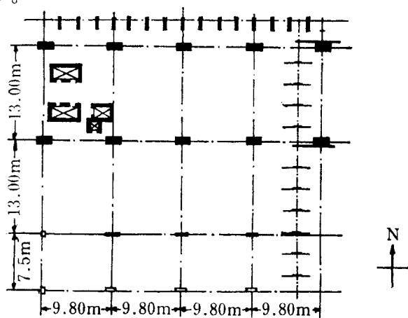
(a)平面图(1)
