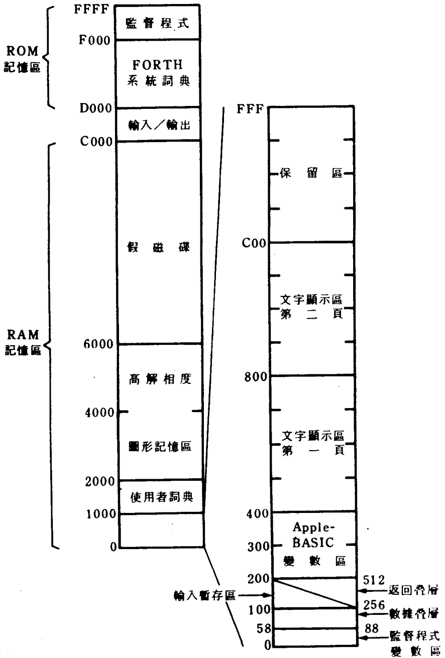
圖 1-1 Apple-FORTH 記憶區分圖
